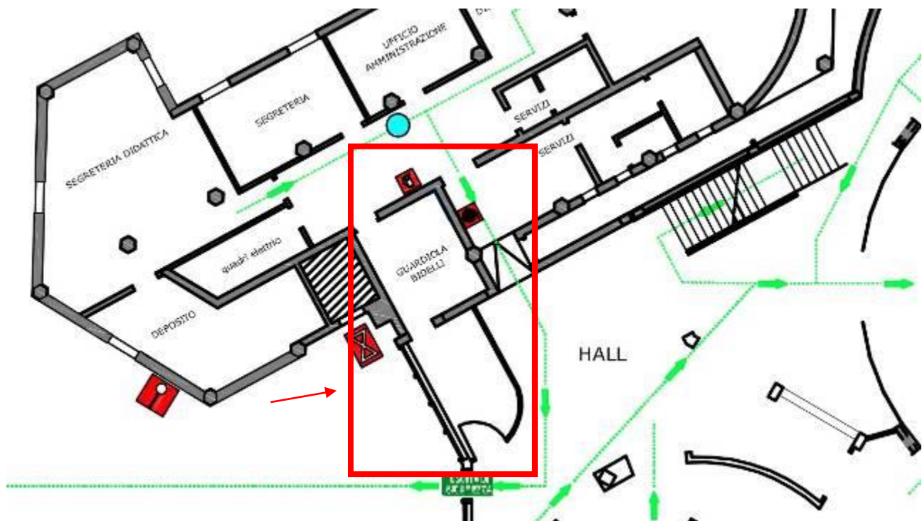
Stralcio piano terra planimetria di emergenza – viene evidenziata in rosso la zona dell’atrio principale dove si colloca il “centro delle emergenze”.
